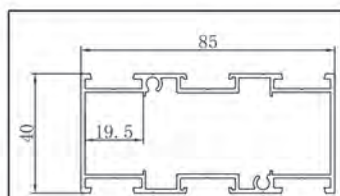
NAME CODE DOOR PREMETER1.4 F8502
